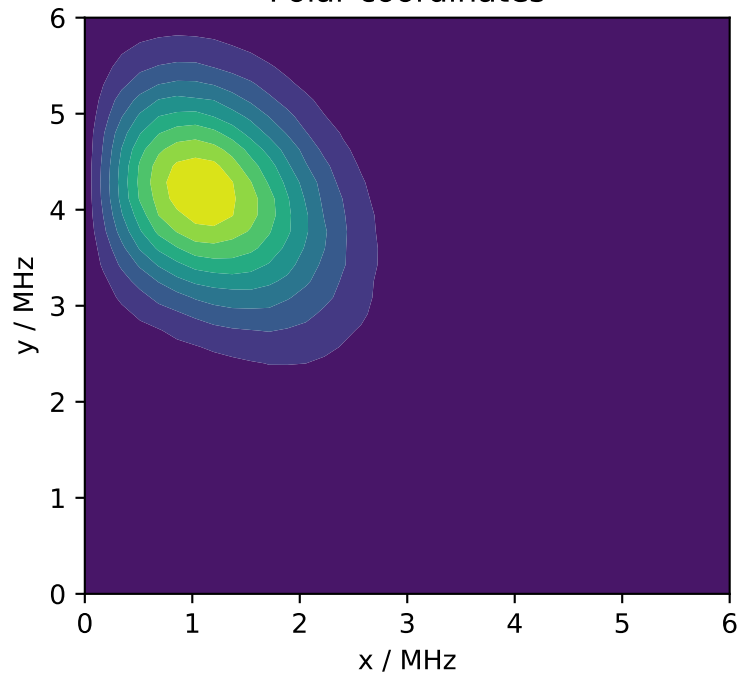
Polar coordinates
